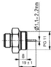
Adaptador PG 11
